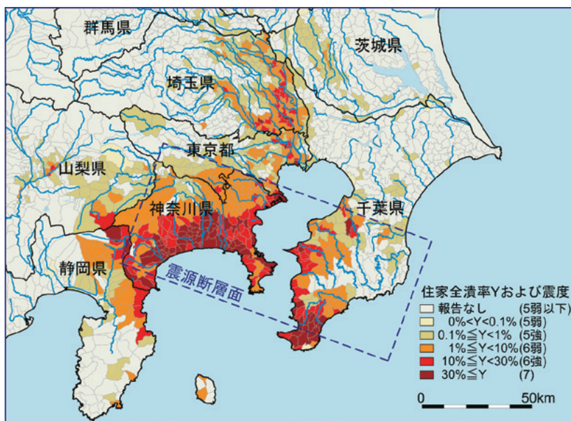
図 1 関東大震災における住家全潰率から評価した震度分布と震源断層の位置（武村, 2003）。
