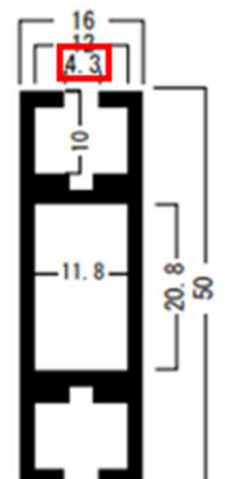
パネル上部(ビーム)の溝の幅:4.3mm
